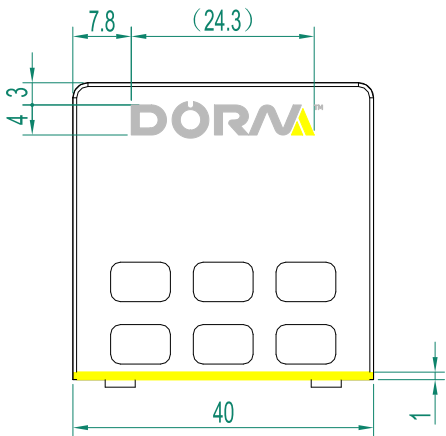
丝印图1(位置)
