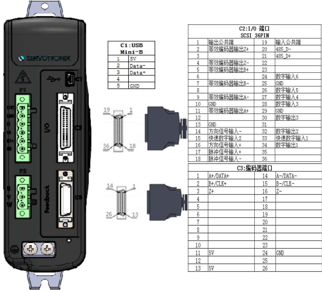
图 4-10 CDHDE-4D52AAP 控制板引脚分配
