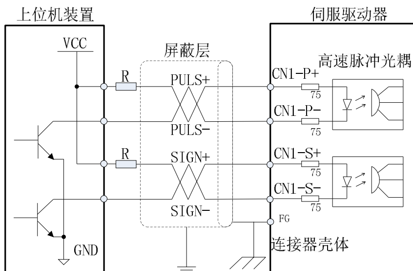
b) 上位机为集电极开路输出，且提供 5VDC、12VDC、24VDC 信号电源时，连接方式 2
