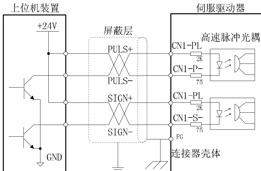
b) 上位机为集电极开路输出，且提供 5VDC、12VDC、24VDC 信号电源时，连接方式 2
